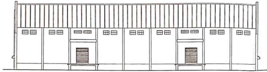
ELEVATION
